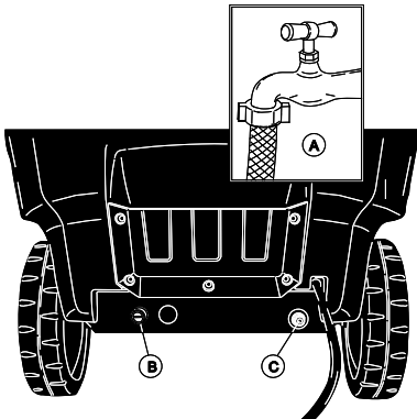
Vesiliitäntä.
